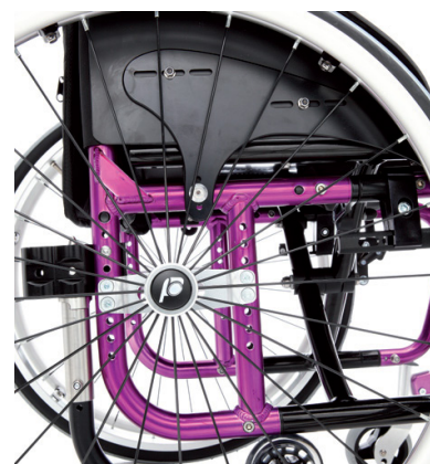
Hinterrahmenversion STANDARD
